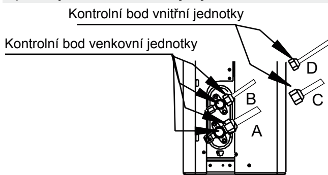
A: Nízkotlaký uzavírací ventil B: Vysokotlaký uzavírací ventil C & D: Vnitřní jednotka světlice matice
